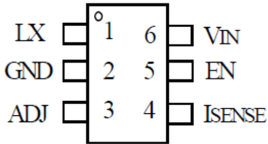
SOT-23-6
