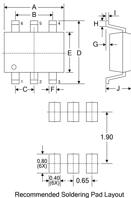
UAT36A03L05: SOT-363
