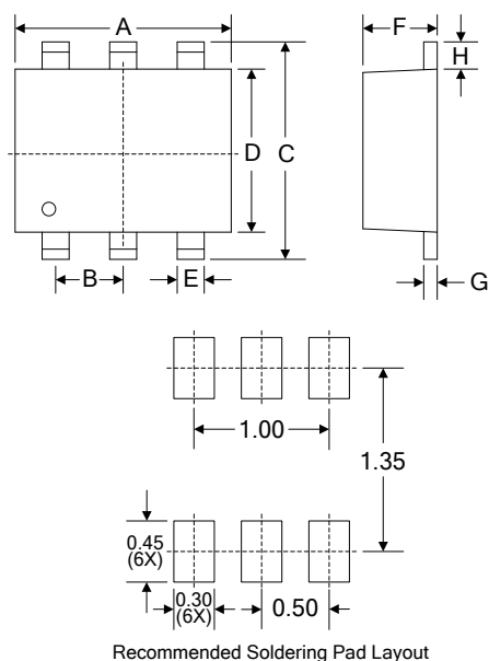
UAT56A03L05: SOT-563
