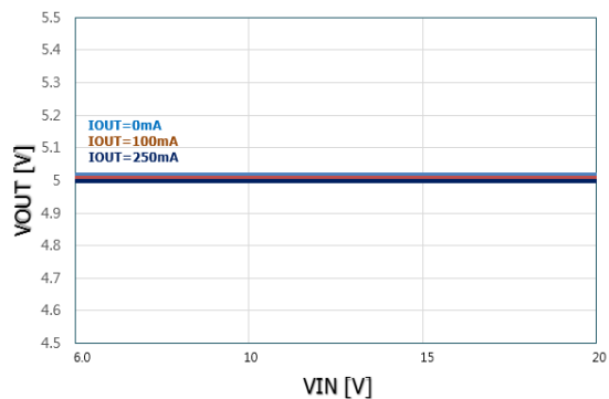
- VOUT vs. IOUT, VIN
