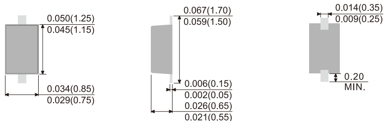
SOD-323HE
