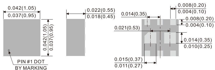
DFN1010-6L
