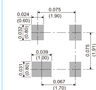
SOT-143
