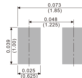
DFN1610-2L
