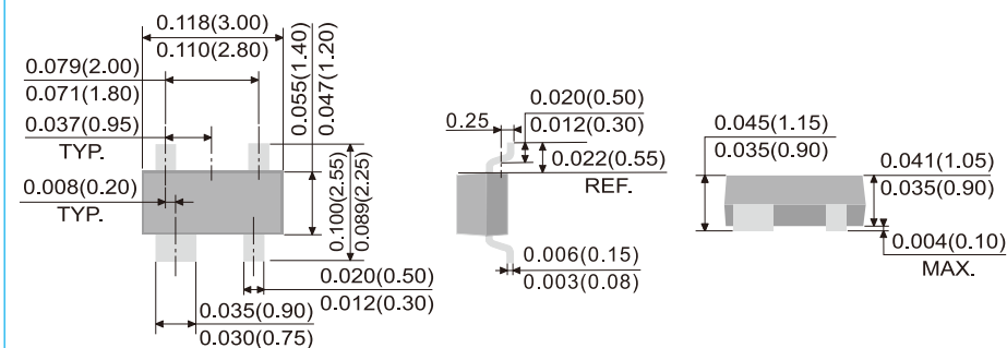
SOT-143
