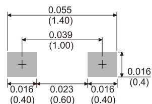
SOD-923
