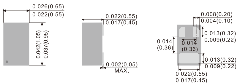
DFN 3L
