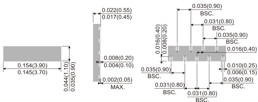
DFN3810-9L
