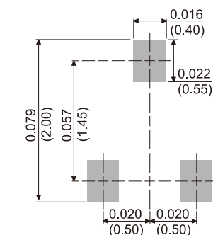
SOT-363
