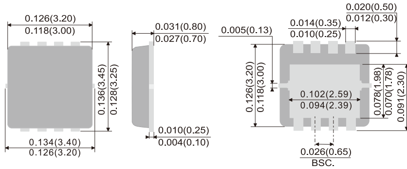
DFN3333B-8L
