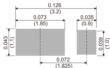
SOD-323HE
