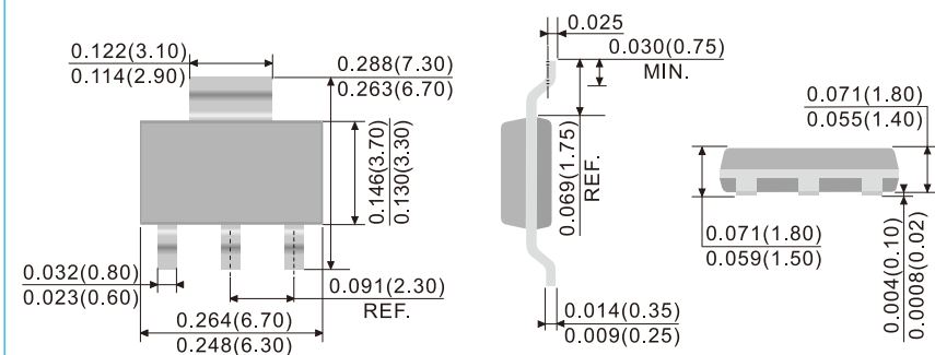
SOT-223
