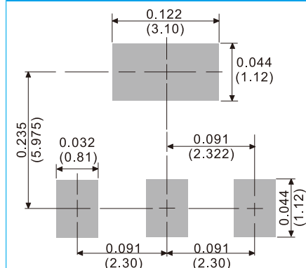
SOT-89
