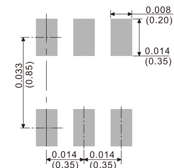
DFN1010-6L
