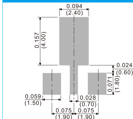
SOT-89
