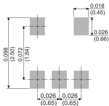
SOT-353
