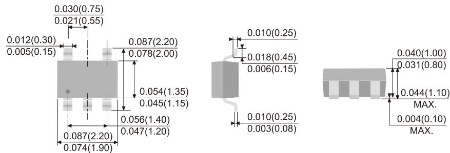
SOT-353
