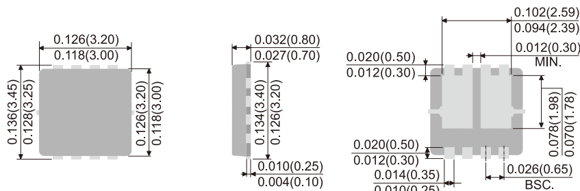
DFN3333B-8L
