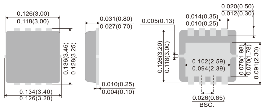
DFN3333-8L
