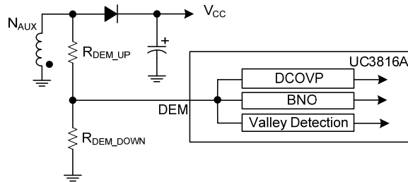
Fig. 6 DEM-Pin Divider
