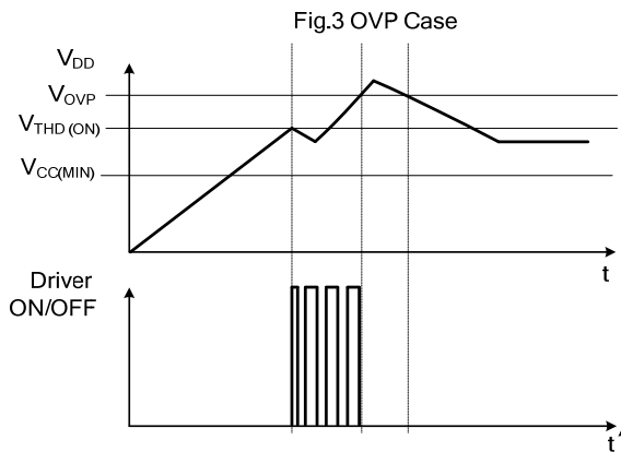
Fig.3 OVP case
