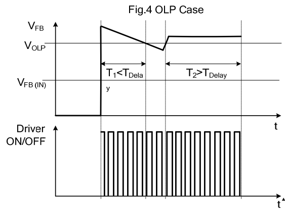
Fig.4 OLP case
